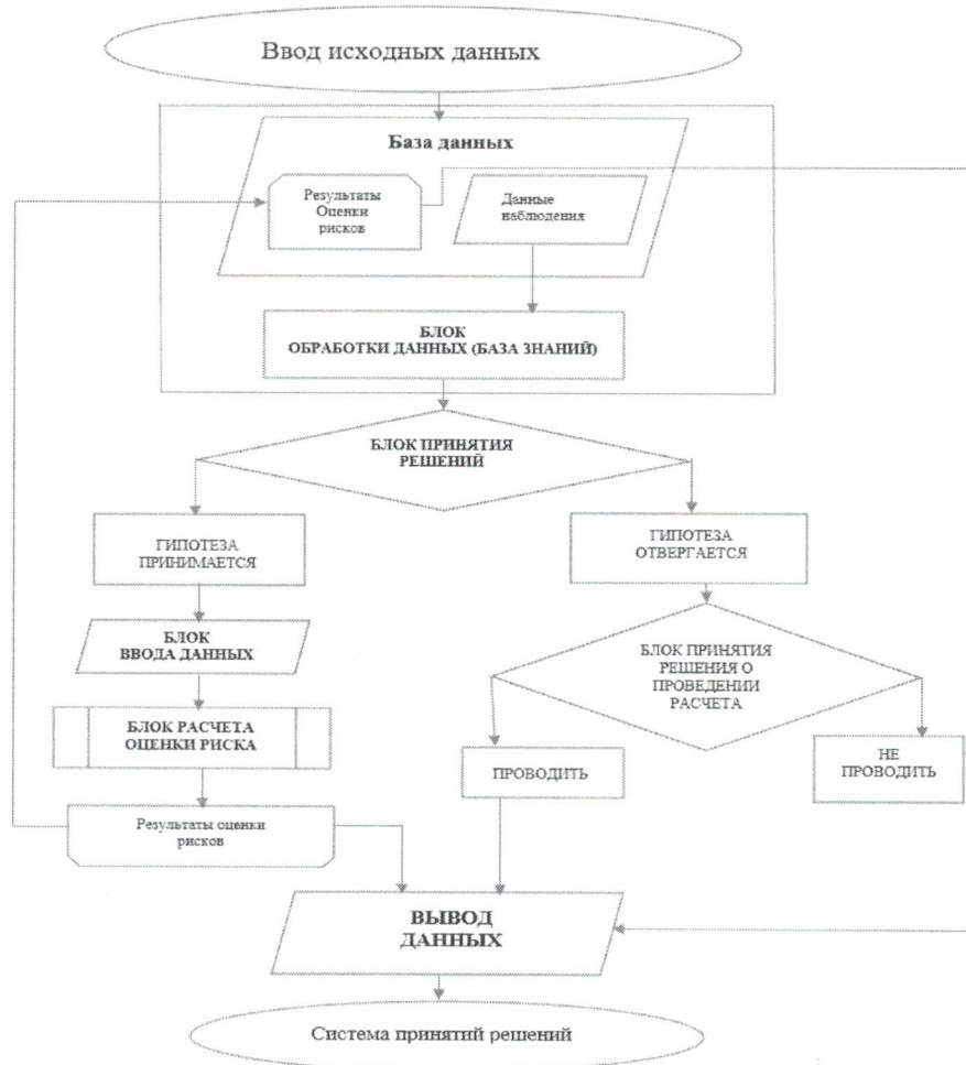
Рис. 13. Блок-схема алгоритма реализации геоинформационной модели оценки гидрометеорологических рисков сельского хозяйства.
