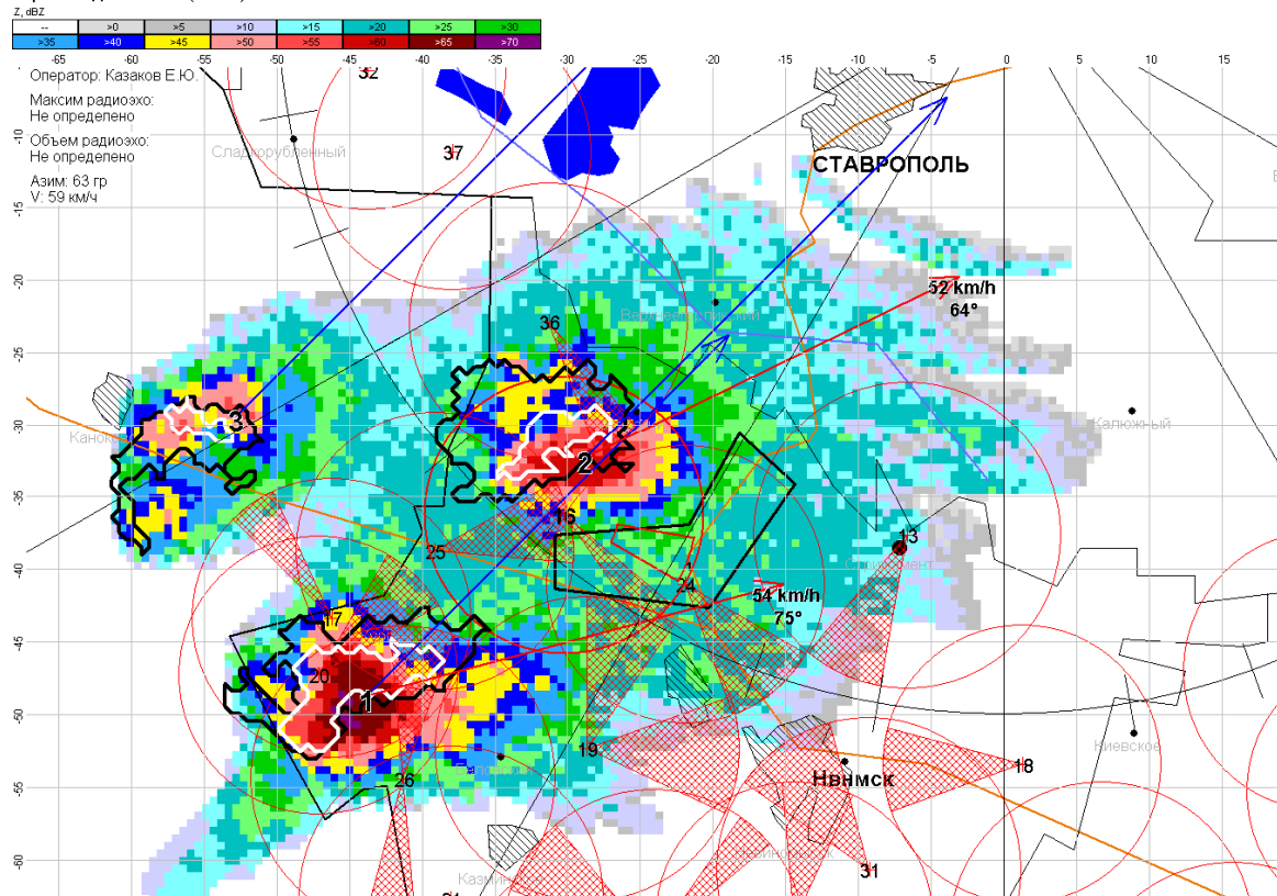
Рис. 4.20 Пример карты двухуровневого сечения градовых облаков 30.08.2008 г. в 19 21 и 19 35 с векторами ведущего потока (синий цвет) и векторами направления и скорости перемещения КЯ (красный цвет).
