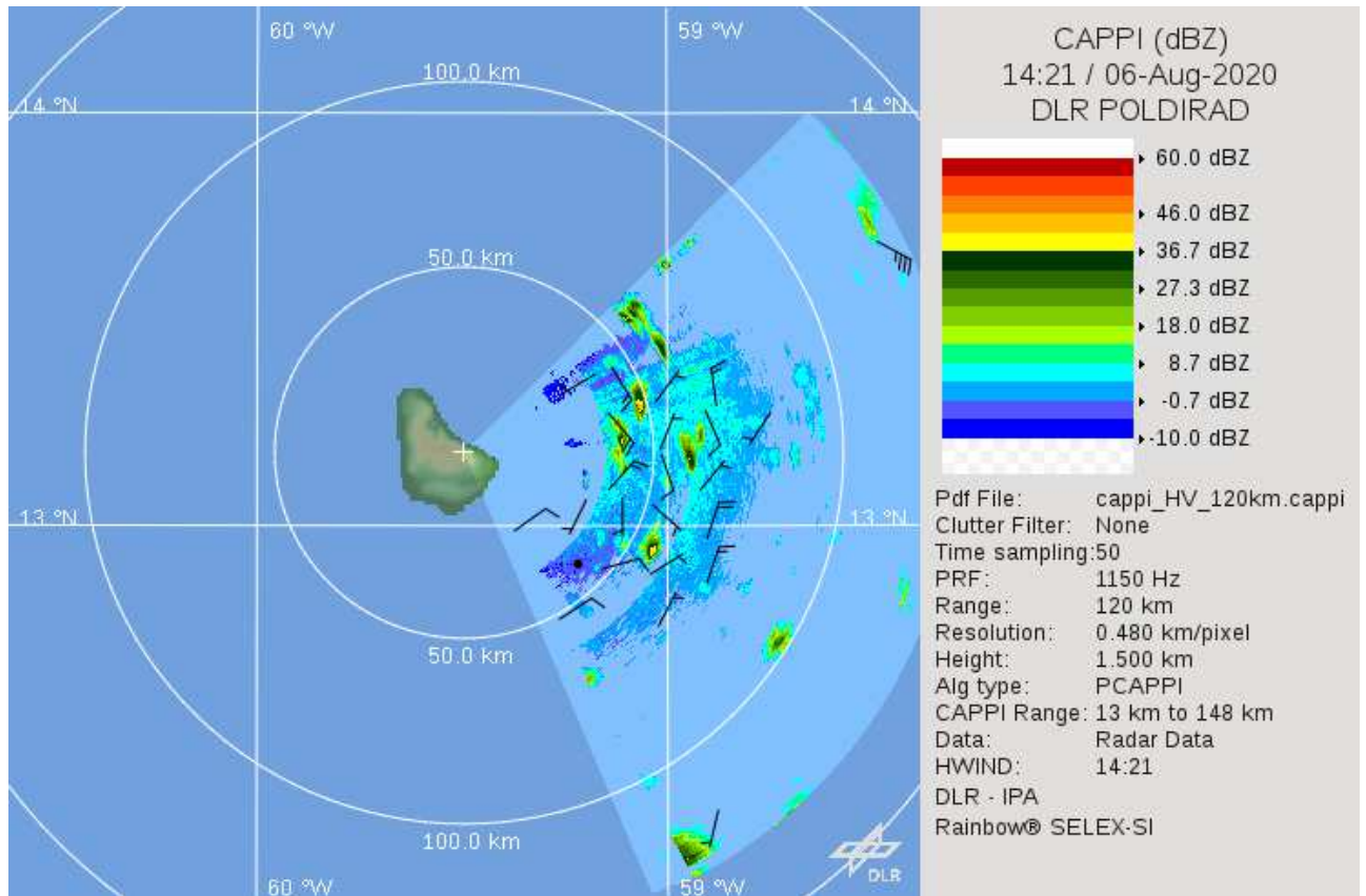
Рис. 1.2 Карта отражаемости на высоте 1.5 км
