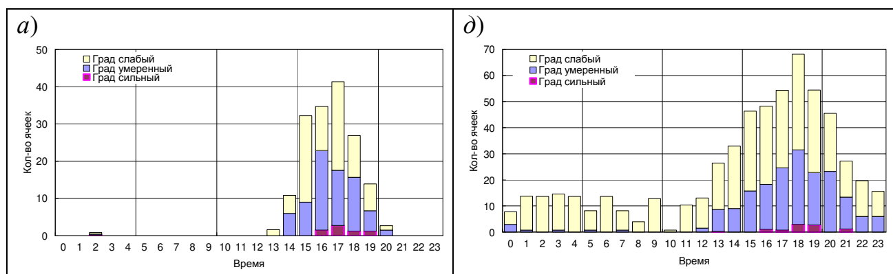
Рис. 4.7 Суточный ход числа градовых КЯ, осредненный по всем месяцам сезона: а) 2002 г., б) 2003 г., в) 2004 г., з) 2005 г., д) 2006 г., е) 2007 г., и) 2008 г.
