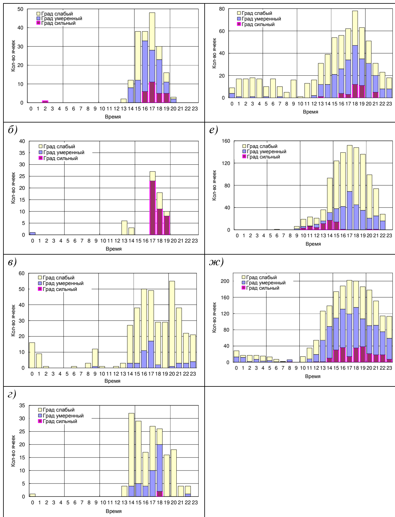
Рис. 4.9 Суточный ход повторяемости КЯ в июне: а) в 2002 г., б) в 2003 г., в) в 2004 г., г) в 2005 г., д) в 2006 г., е) в 2007 г., ж) в 2008 г., соответственно.
