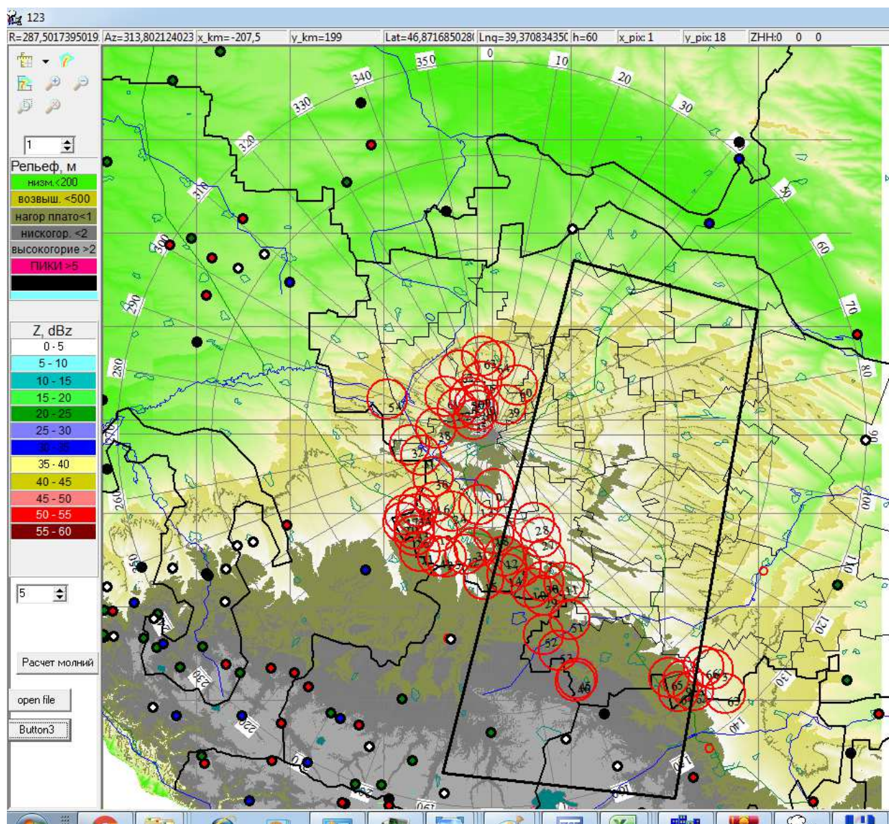
Рис.4.32 Распределение максимальных положительных и отрицательных зарядов в канале молнии, за 2009-2019 гг.
