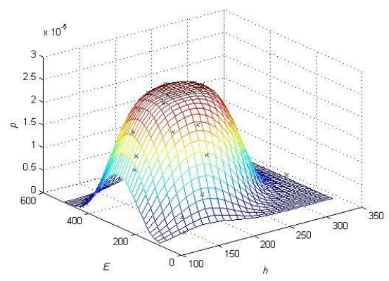
Рисунок 4.6 – Пост Rahim Abad : а – гистограмма годовых значений испарения и слоя стока, б – эллипсы рассеивания, в – трехмерная плотность вероятности; пост Dorud Tire : г – гистограмма годовых значений испарения и слоя стока, д – эллипсы рассеивания, ж – трехмерная плотность вероятности.
