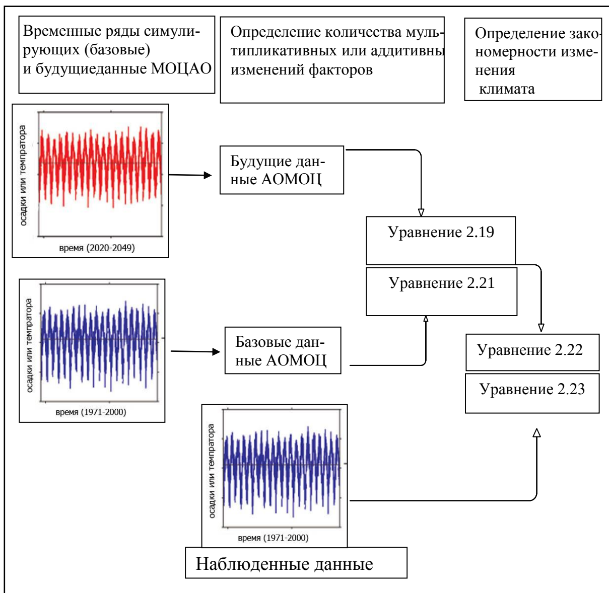
Рисунок 2.5– Схема метода МОТП.
