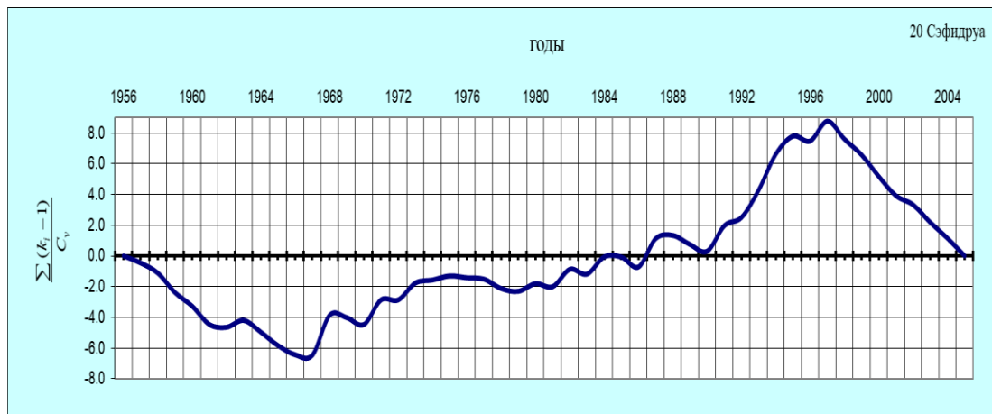
Рисунок А.5 – Разностно-интегральная кривая Mahneshan р. Сефидруд.
