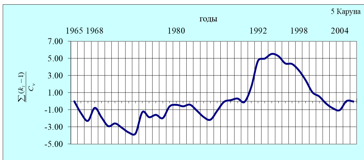
Рисунок 1.16 – Разностно-интегральная кривая Kohe Sokhte р. Карун.
