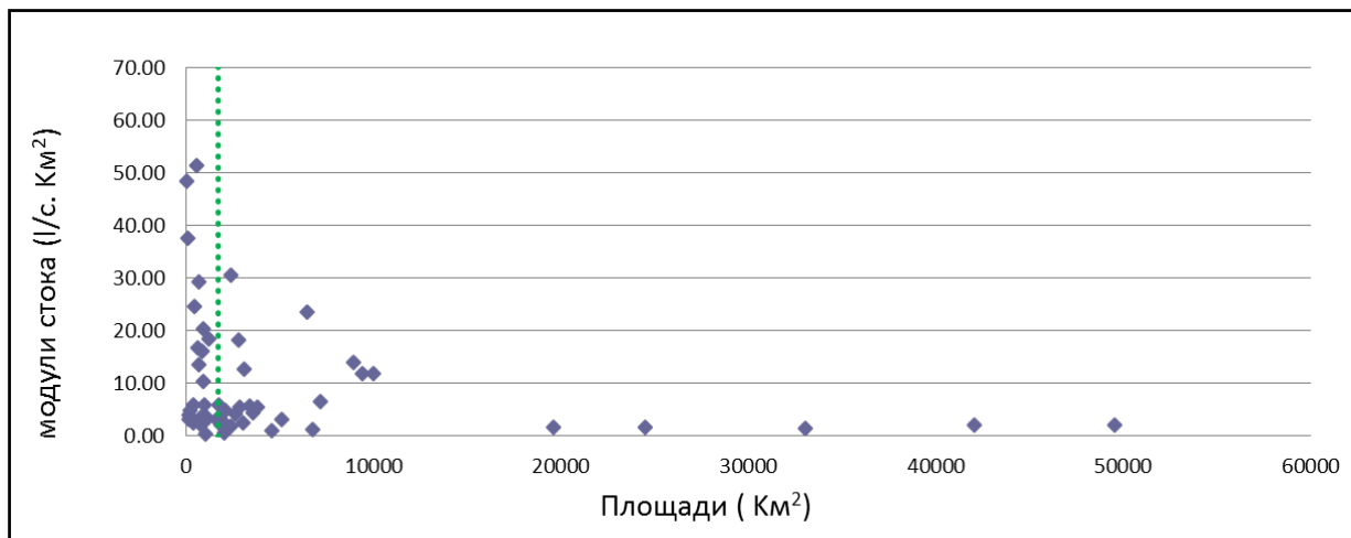
Рисунок 1.13 – Редукционная зависимость для бассейнов рек Сефидруд и Карун.
