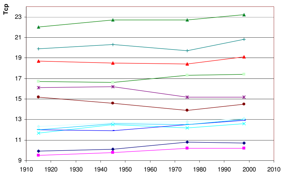
Рисунок 4.3 – Значимые изменения климатических норм температур января на метеостанциях Аравийского полуострова.
