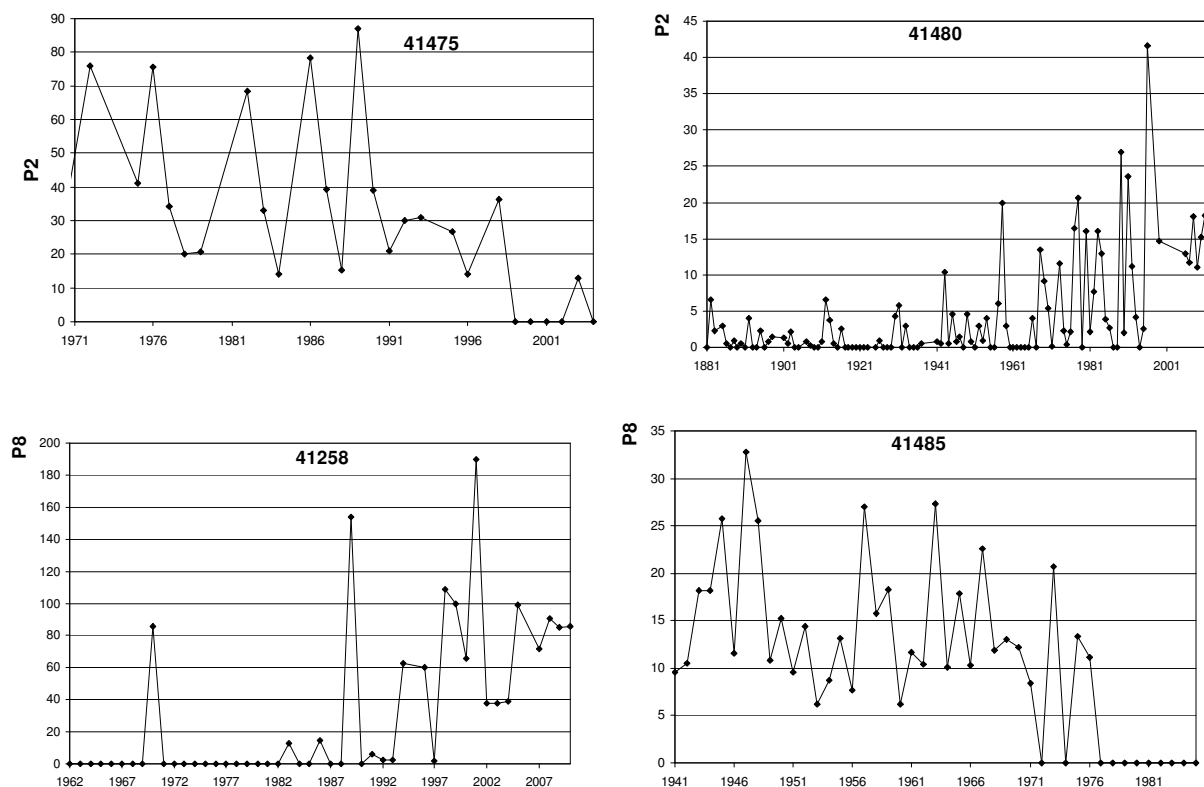
Рисунок 3.10 – Нестационарных ряды месячных сумм осадков на метеостанциях Аравийского полуострова.
