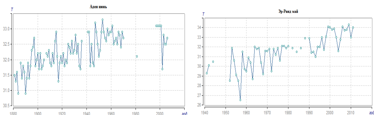
Рисунок 2.6 – Примеры рядов наблюдений, нестационарных по средним значениям.
