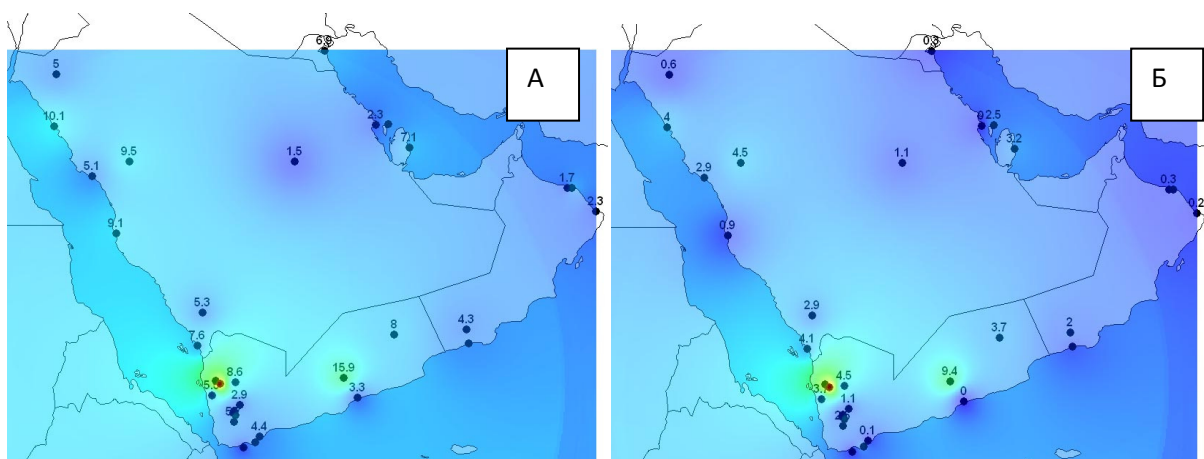
Рисунок 3.11 – Пространственная модель отклонений от нестационарности \Delta в % для осадков января и модели: А – ступенчатых изменений, Б – линейного тренда.
