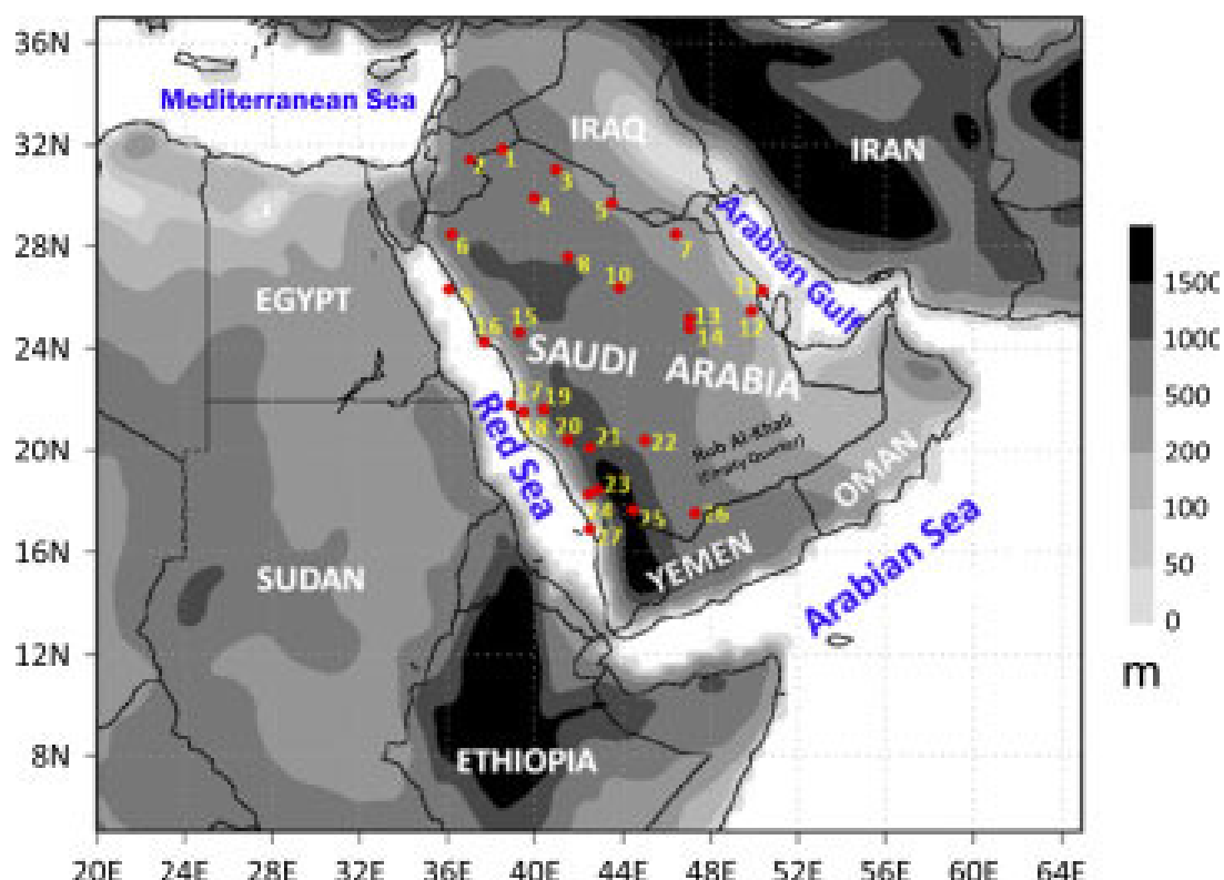
Рисунок 1.4 – Гипсографическая карта Аравийского полуострова с пунктами наблюдений (красные точки) и их номерами.
