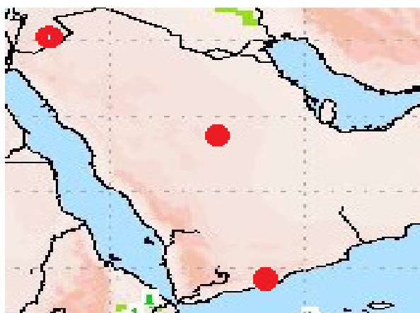
Рисунок 1.10 – Расположение трех выбранных метеостанций на территории Аравийского полуострове (с севера на юг: Иордания, Эр-Риад, Аден).
