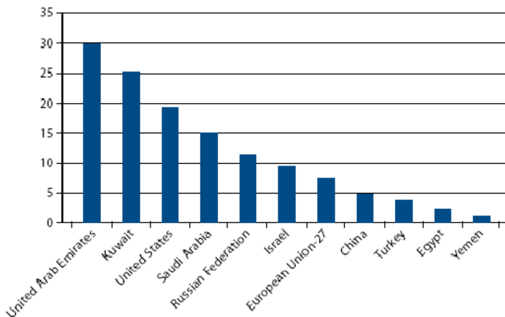
Рисунок 1.6 – Вклад отдельных стран Ближнего Востока и других стран мира в эмиссию углекислого газа.
