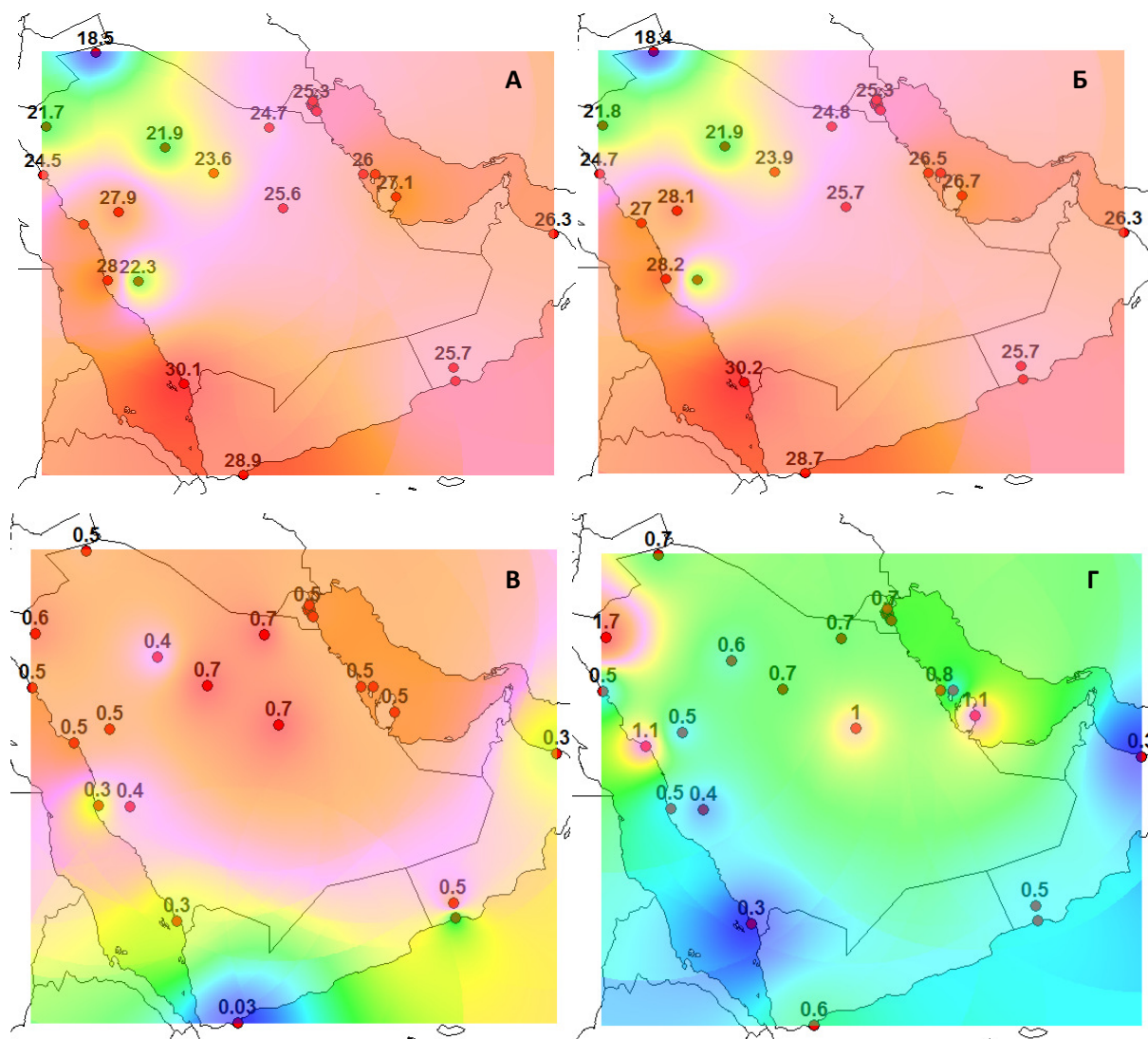
Рисунок 4.6 – Пространственная изменчивость параметров распределения среднегодовых температур на Аравийском полуострове (А, Б - норма темпе-
