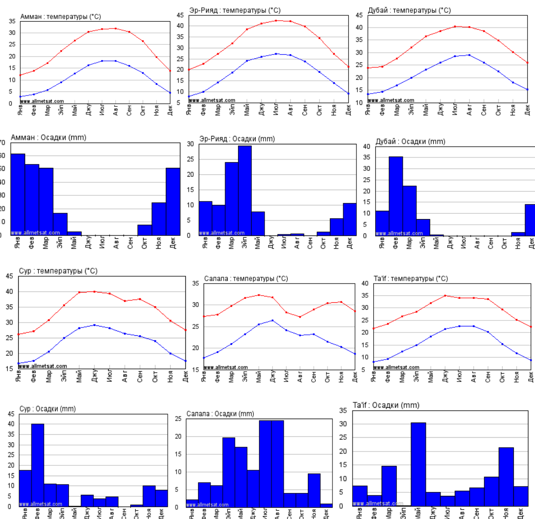
Рисунок 1.2 – Внутригодовые распределения температур воздуха и осадков на метеостанциях Аравийского полуострова.
