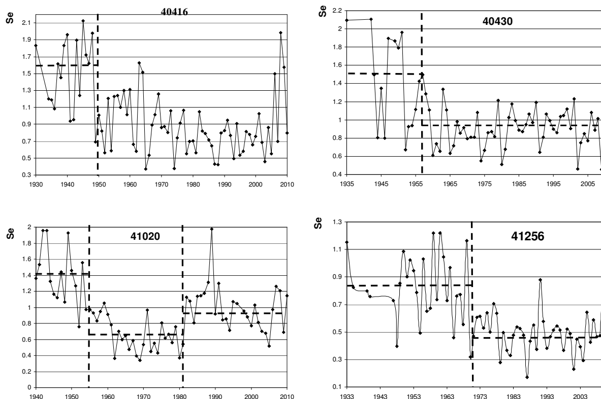
Рисунок 3.8 – Нестационарные ряды параметра Se внутригодовой функции температуры воздуха.
