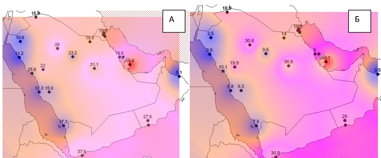
Рисунок 3.6 – Пространственная модель отклонений от нестационарности \Delta в % для среднегодовой температуры воздуха и модели: А – ступенчатых изменений, Б – линейного тренда.
