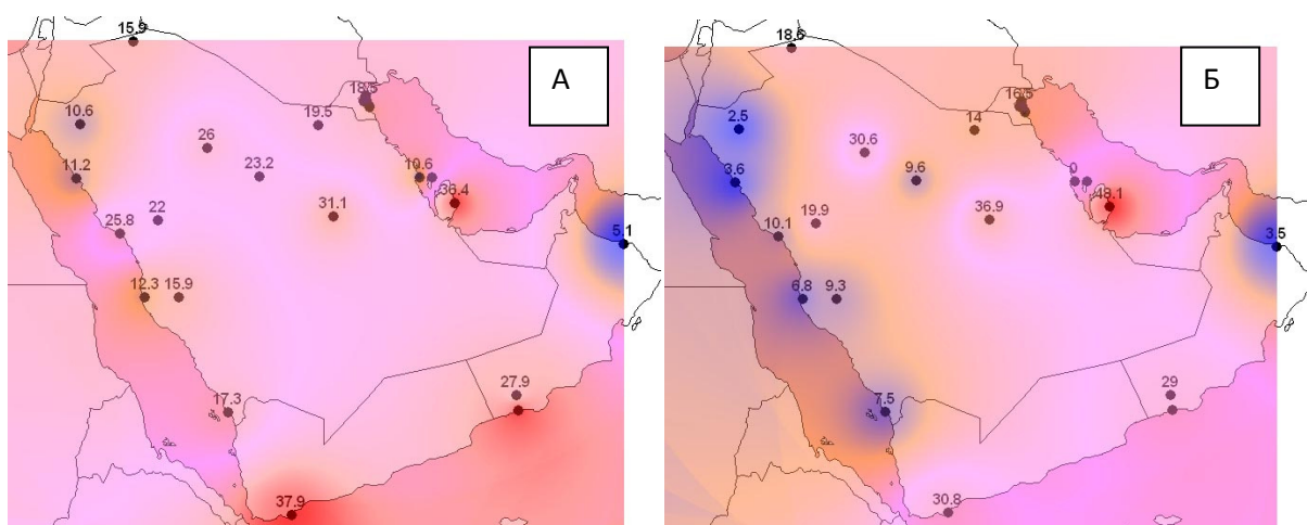
Рисунок 3.9 – Пространственная модель отклонений от нестационарности \Delta v % для параметра Se и модели: А – ступенчатых изменений, Б – линейного тренда.
