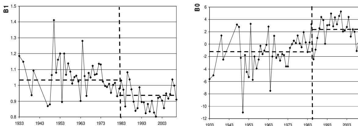
Рисунок 3.7 – Нестационарные временные ряды коэффициентов B1 и B0 функции внутригодовых колебаний на метеостанции Сиб.
