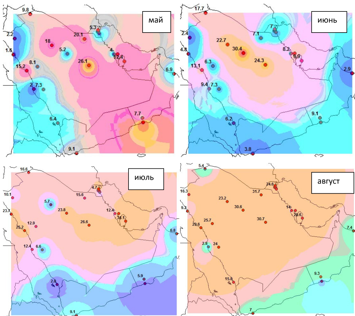
Рисунок 3.2 – Пространственная модель отклонений от нестационарности \Delta_{стун} в % для среднемесячной температуры мая, июня, июля и августа.
