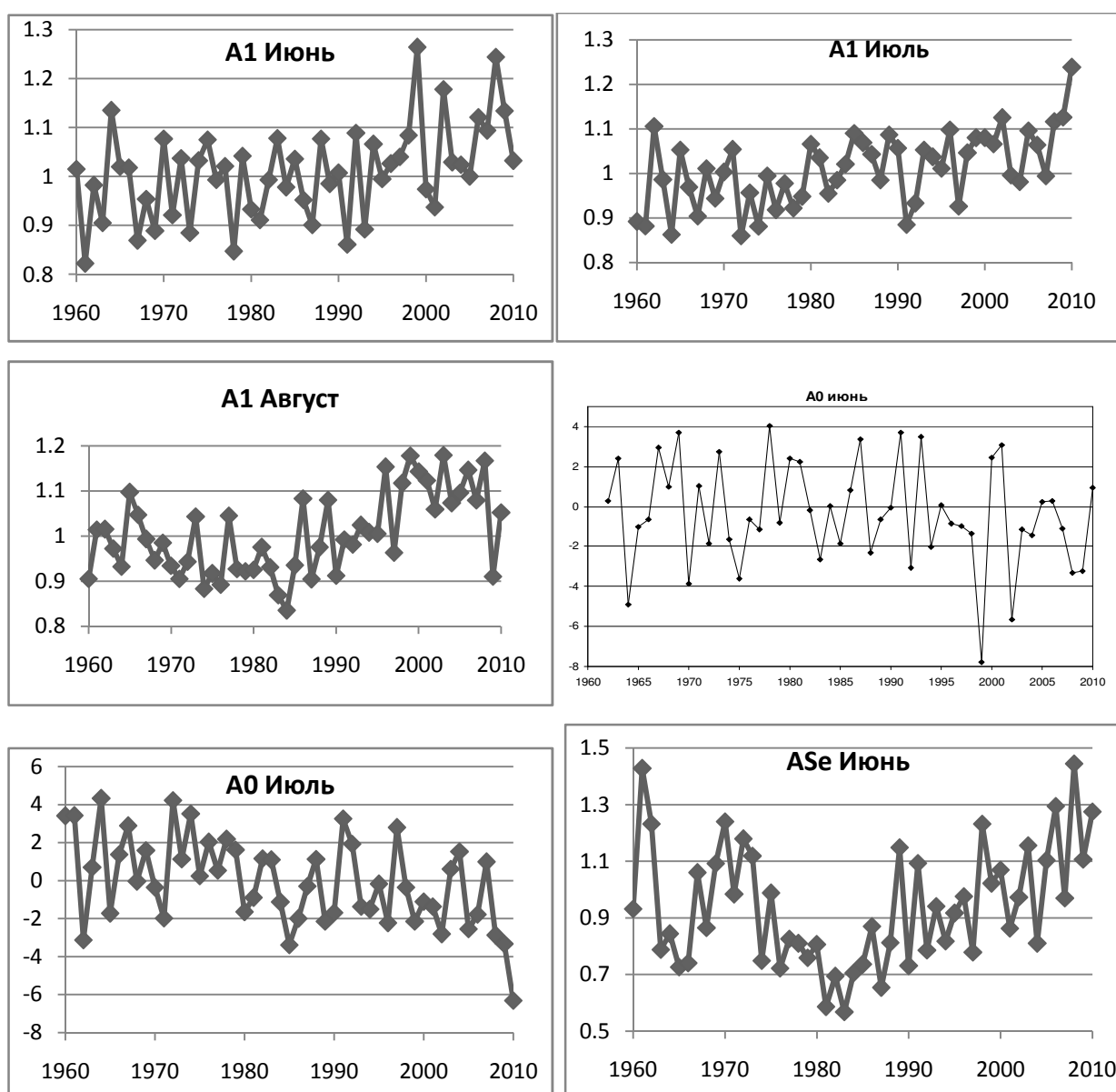
Рисунок 4.10 – Нестационарные ряды коэффициентов A1, A0 и ASe для температур летних месяцев на Аравийском полуострове.
