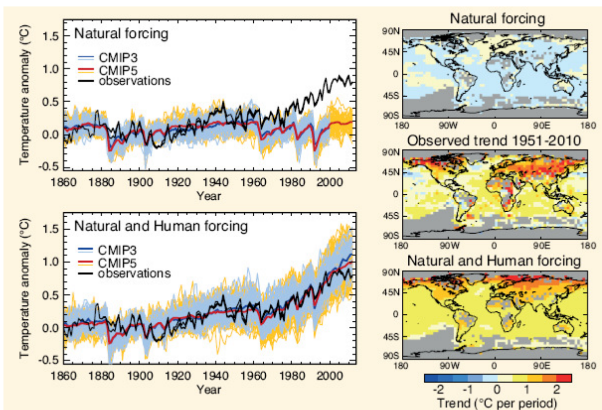
Рисунок 1.3 – Разделение колебаний глобальной температуры и пространственного распределения трендов на естественные и антропогенные составляющие.
