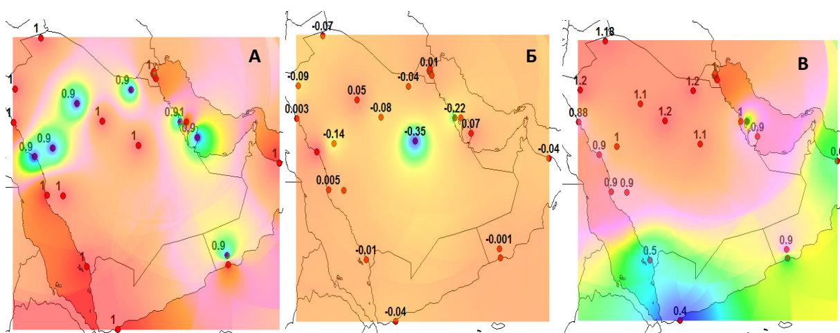
Рисунок 4.7 – Пространственная изменчивость норм коэффициентов функции внутригодовых колебаний, где А – коэффициент B_1 , Б – коэффициент B_0 , В – параметр Se за весь период наблюдений.
