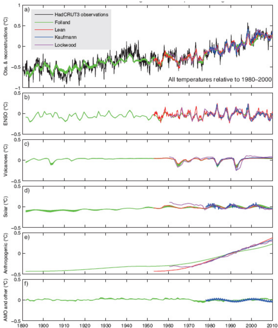
Рисунок 1.2 – Аномалии колебания глобальной температуры и основных формирующих ее факторов.
