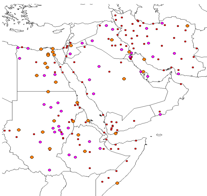
Рисунок 2.3 – Распределение метеостанций по продолжительности наблюдений за температурой воздуха (наименьшие окружности n < 50 лет, средние 50 < n < 70 лет и большие – n > 70 лет).
