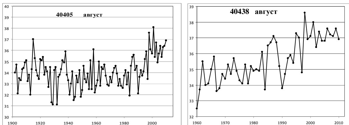
Рисунок 3.4 – Примеры нестационарных рядов среднемесячных температур воздуха на станциях Аравийского полуострова.
