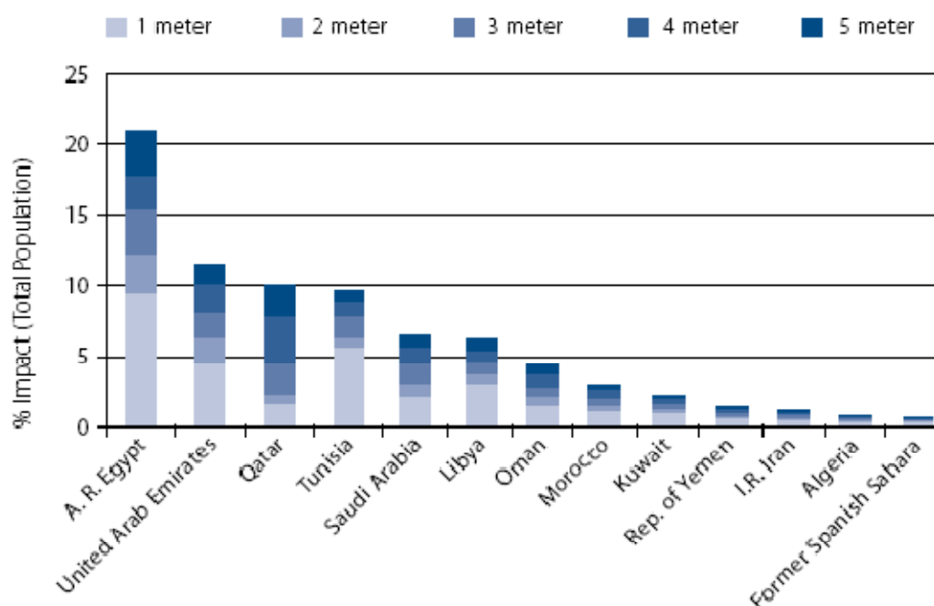
Рисунок 1.7 – Влияние повышения уровня Мирового океана на 1 м, 2 м, 3 м, 4 м и 5 м на население отдельных стран Аравийского полуострова и Северной Африки (в % от общего числа жителей).
