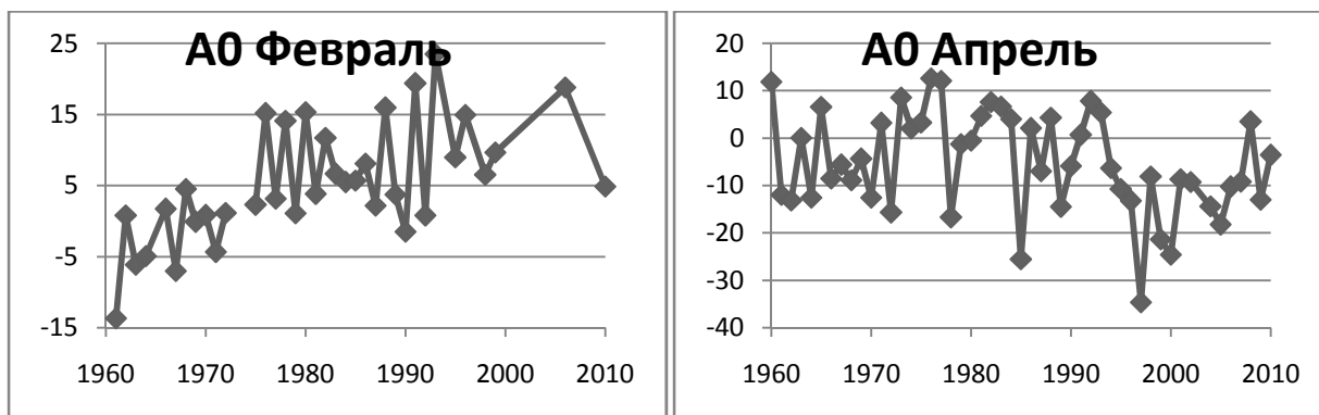
Рисунок 4.11 – Нестационарные ряды коэффициентов A , и A_0 для осадков на Аравийском полуострове.
