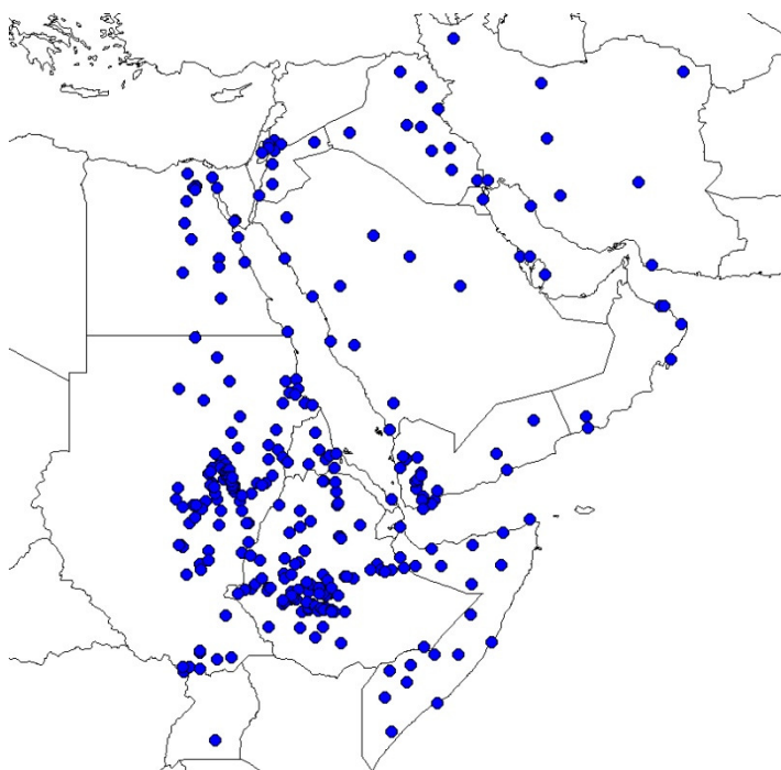
Рисунок 2.2 – Расположение метеостанций региональной БД осадков.
