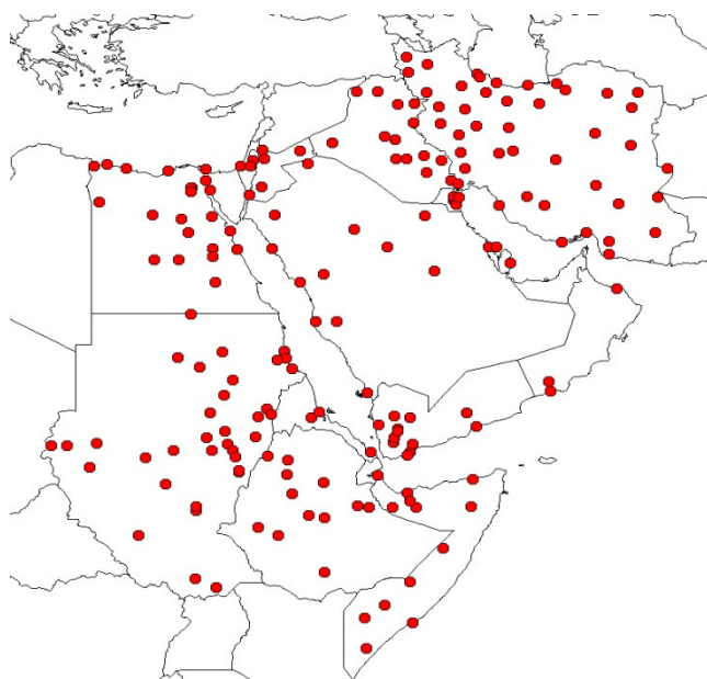
Рисунок 2.1 – Расположение метеостанций региональной БД температур воздуха.
