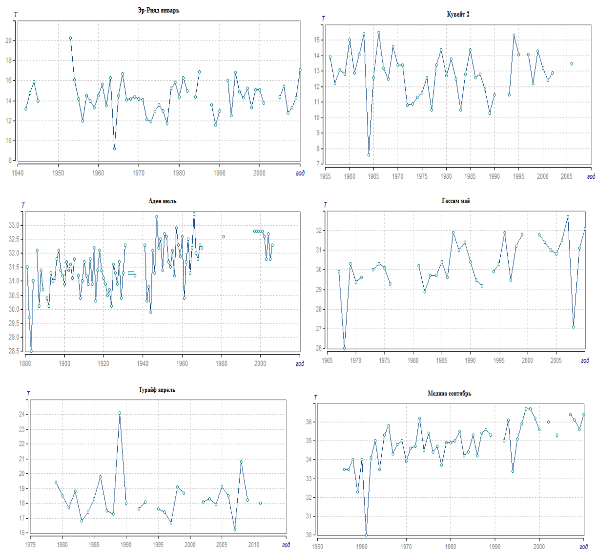
Рисунок 2.5 – Примеры неоднородных экстремумов в рядах среднемесячных температур воздуха.
