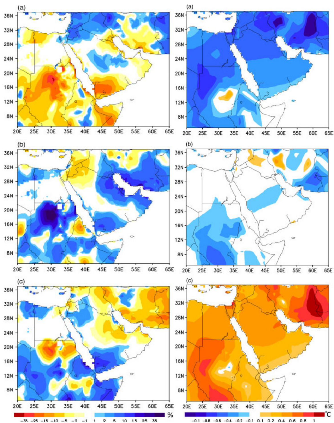
Рисунок 1.5 – Пространственные распределения аномалий осадков (слева) и среднегодовых температур (справа) за три отдельных десятилетия (сверху вниз): 1980-1989 гг., 1990-1999 гг., 2000-2009 гг. по отношению к базовому периоду 1979-2009 гг.
