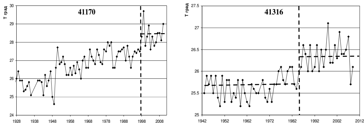
Рисунок 3.5 – Примеры нестационарных рядов среднегодовых температур воздуха на станциях Аравийского полуострова.
