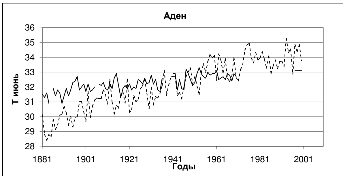
Рисунок 1.11 – Хронологические графики наблюдаемой (сплошная линия) и смоделированной (пунктирная линия) температуры июня по метеостанции Аден за период с 1881 по 2000 гг. для сценария 2 и модели центра метеорологических национальных исследований Франции.
