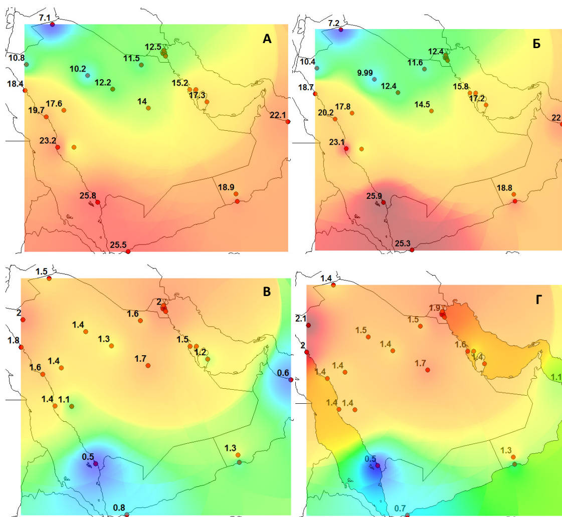
Рисунок 4.2 – Пространственная изменчивость параметров распределения температур января на Аравийском полуострове (А, Б - норма температуры за период ВМО и за весь период наблюдений; В,Г - среднее квадратическое отклонение за период ВМО и за весь период наблюдений).
