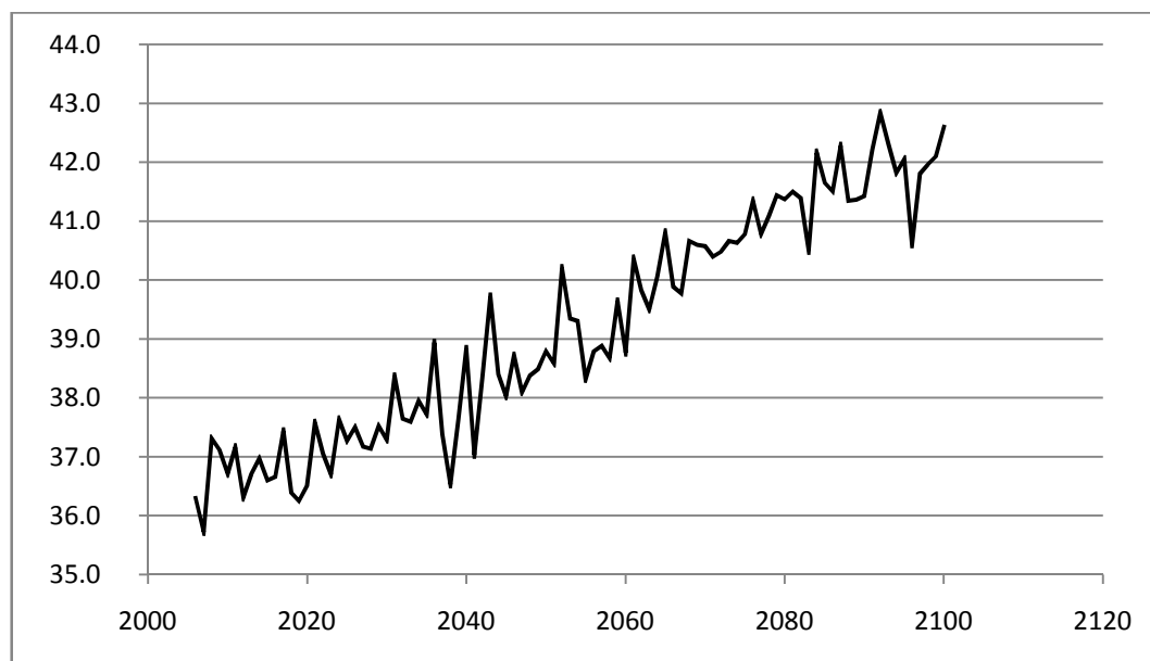
Рисунок 1.13 – Модельные значения температуры июня для метеостанции Аден по сценарию 1 и модели канадского центра по климатическому моделированию и анализу (2014 – 2100 гг).
