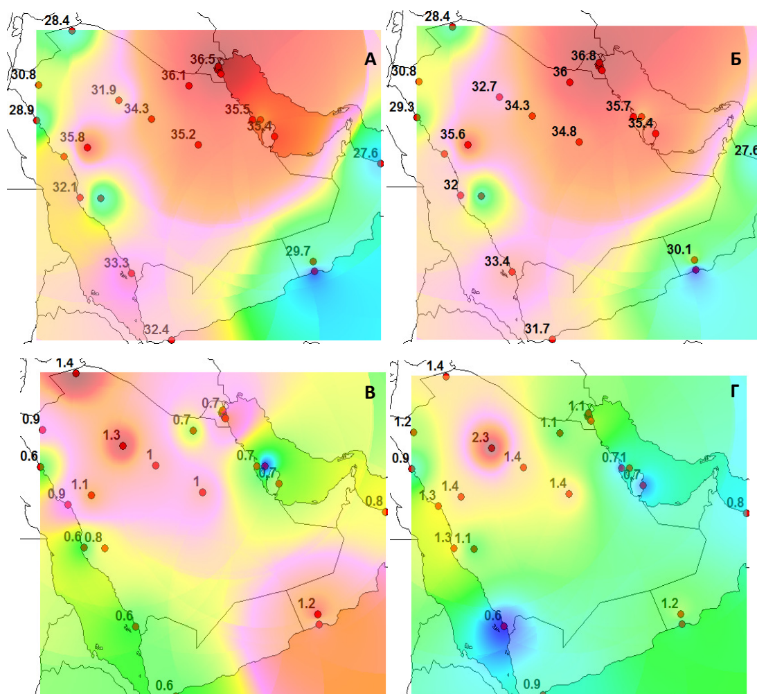
Рисунок 4.4 – Пространственная изменчивость параметров распределения температур июля на Аравийском полуострове (А, Б - норма температуры за период ВМО и за весь период наблюдений; В,Г - среднее квадратическое отклонение за период ВМО и за весь период наблюдений).
