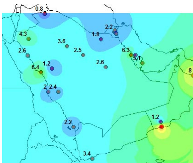
Рисунок 3.1 – Пространственная модель отклонений от нестационарности \Delta_{стун} в % для среднемесячной температуры января.
