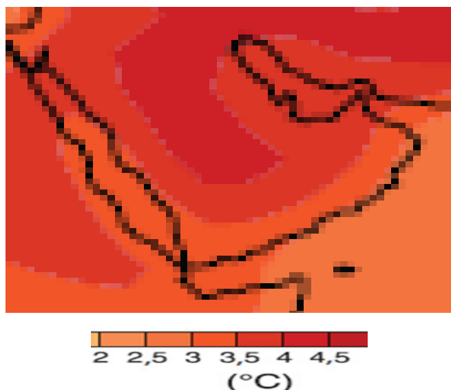
Рисунок 1.8 – Проекция изменений приземной температуры на конец XXI столетия (2090-2099гг.). На карте показана усредненная проекция нескольких моделей МОЦАО для сценария A1B СДСВ. Все температуры показаны по отношению к периоду 1980-1999 гг.
