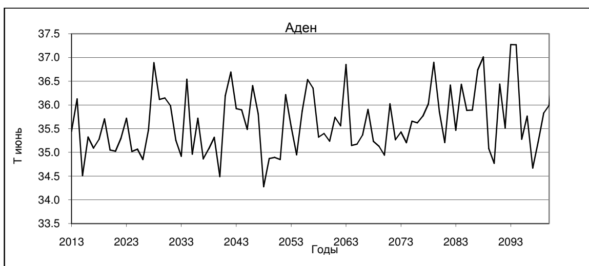
Рисунок 1.12 – Модельные значения температуры июня для метеостанции Аден по сценарию 2 и модели центра метеорологических национальных исследований Франции (2014-2100 гг.).
