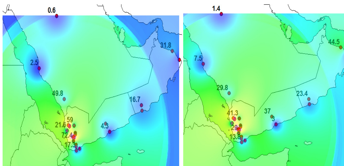
Рисунок 4.9 – Пространственное распределение норм и стандартных отклонений осадков августа на Аравийском полуострове, полученных по данным за многолетний период (левый рисунок – нормы осадков, правый – средние квадратические отклонения).
